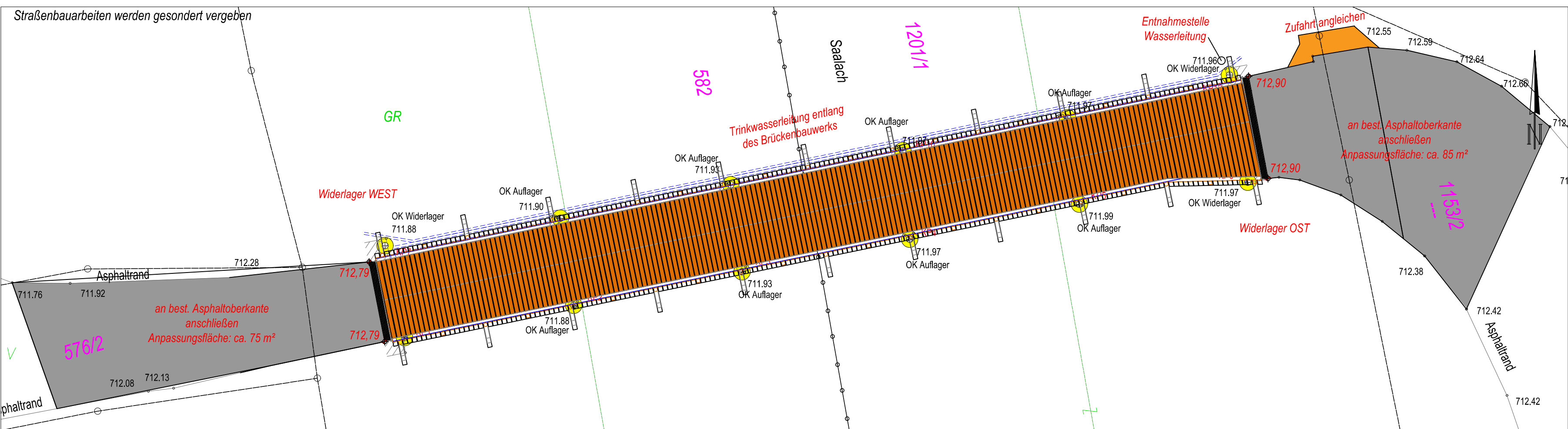
LAGEPLAN STRASSENBAU M1:200
